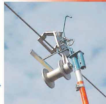
Herramienta elevadora de cables de doble punta 18110812
